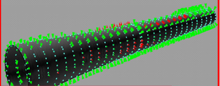
Rotorblattsektion (Stahl) Soll/Ist-Vergleich
