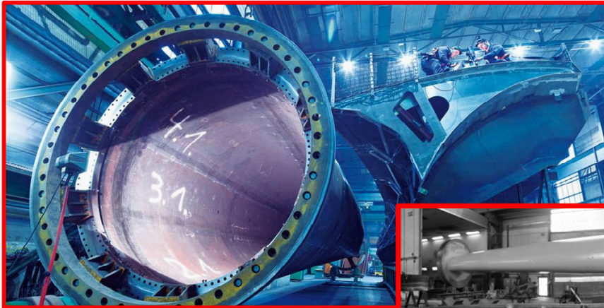
Rotorblattfertigung bei MAM Magdeburg
