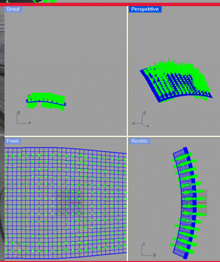
Warmverformte Stahlplatte (Freiform) – Soll/Ist Vergleich
