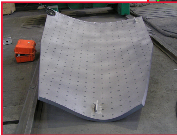
Warmverformte Stahlplatte (Freiform) – Soll/Ist Vergleich
